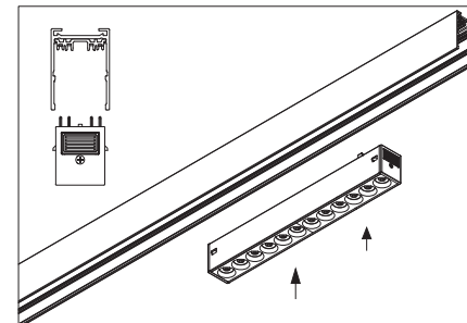
Накладной/Подвесной Арт. 135299; 135300; 135301
